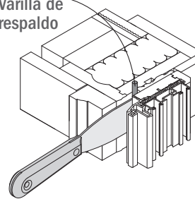
Tilt-Wash Double-Hung Insert Window Ventana de inserción de doble guillotina inclinable para limpieza
