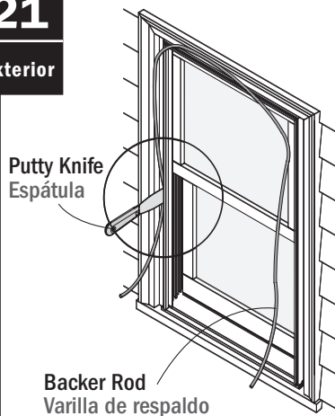
Backer Rod Varilla de respaldo
